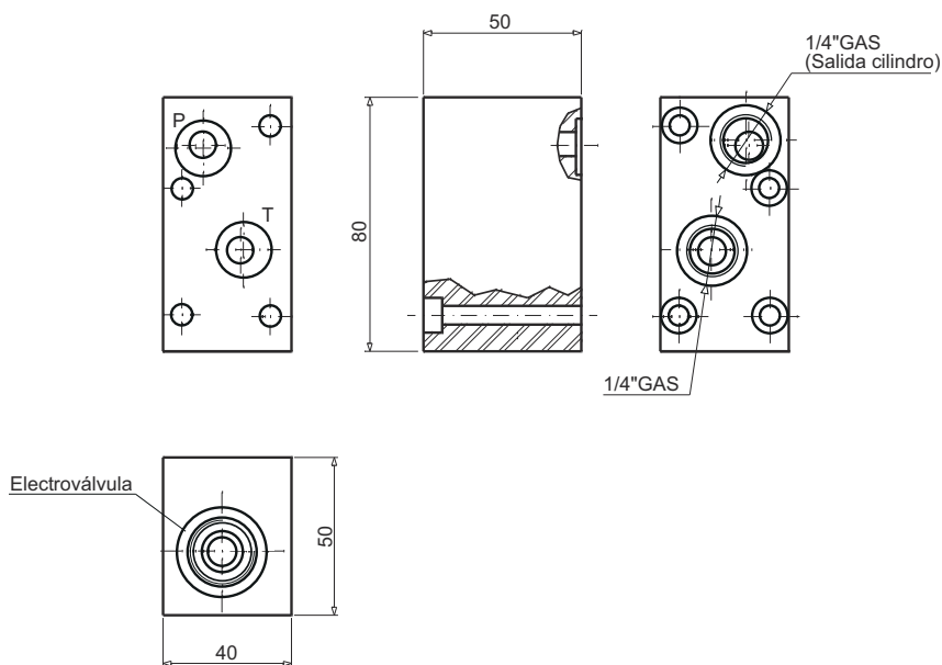
Elevación 2 velocidades descenso Lift 2 speed
