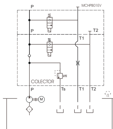
Elevación 2 velocidades descenso Lift 2 speed
